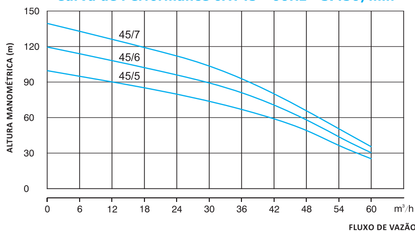
Seleção de Curva - 60Hz
