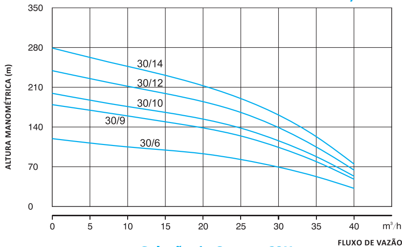
Seleção de Curva - 60Hz
